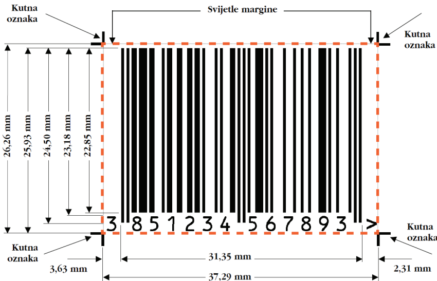
Dimenzije EAN-13 simbola u faktoru uvećanja 1,0
